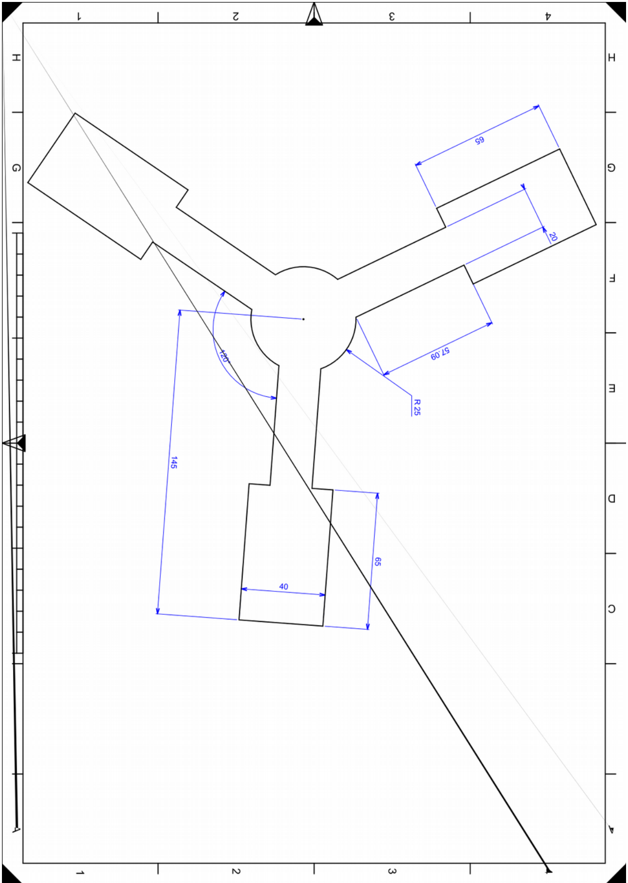
Plan de pièce pour le support pour faire tenir la tête de micro 2 - prévoyez un trou au centre de la pièce pour enfiler le corps du micro
